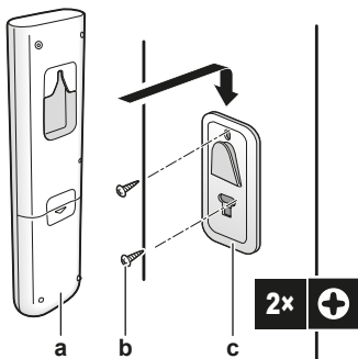
a Uživatelské rozhraní b Šroub c Držák uživatelského rozhraní
